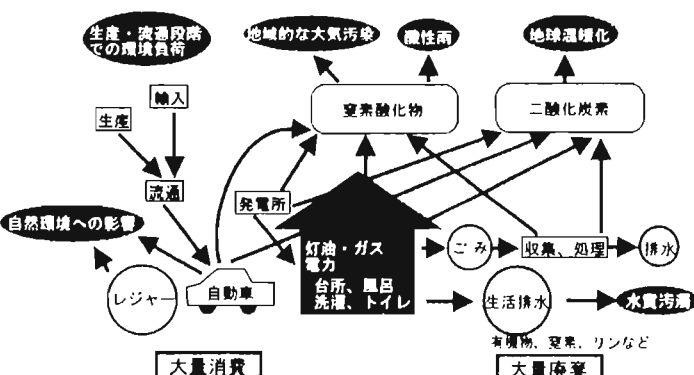
(図2) ライフスタイルと環境負荷(平成6年度環境白書より)
