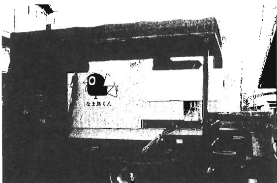
生ごみ分選機で圧搾処理（ペースト化）
