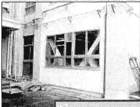
耐震補強された 校舎(高南小学校)
